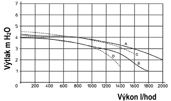
Charakteristiky čerpadel s podlahovou sadou
