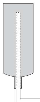
Plnění pomocí lahve bez připojeného sifonu Naplňte tekuté chladivo s lahví vzhůru nohama
