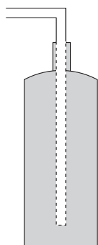
Plnění pomocí lahve s připojeným sifonem Naplňte tekuté chladivo se vzprímenou lahví
