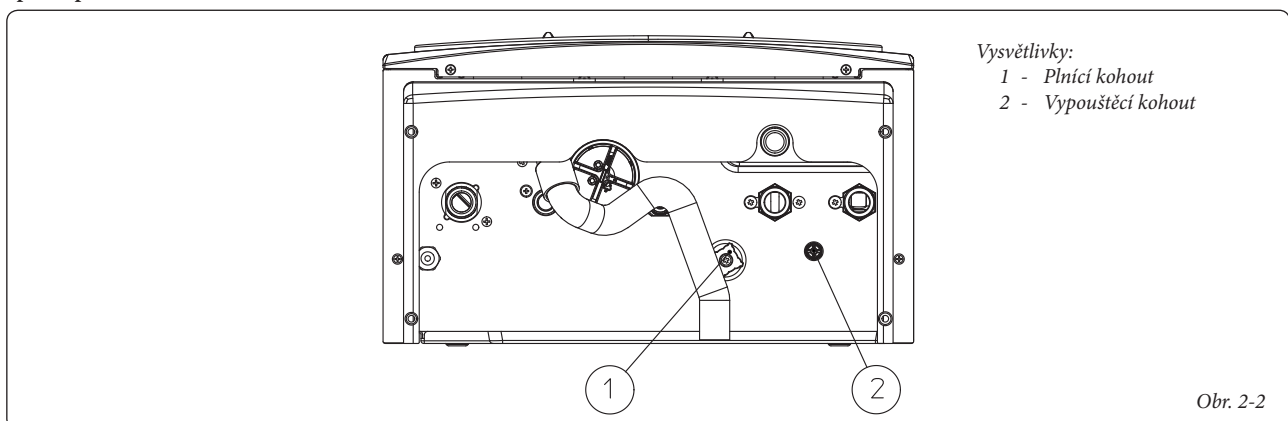
Spodní pohled.
