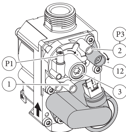
Plynový ventil 8205
