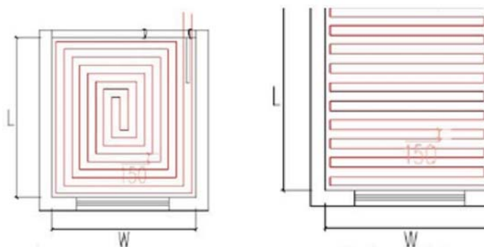
Smyčka ve tvaru čtvercové spirály (šnek, doporučeno) Smyčka ve tvaru meandru (had)
