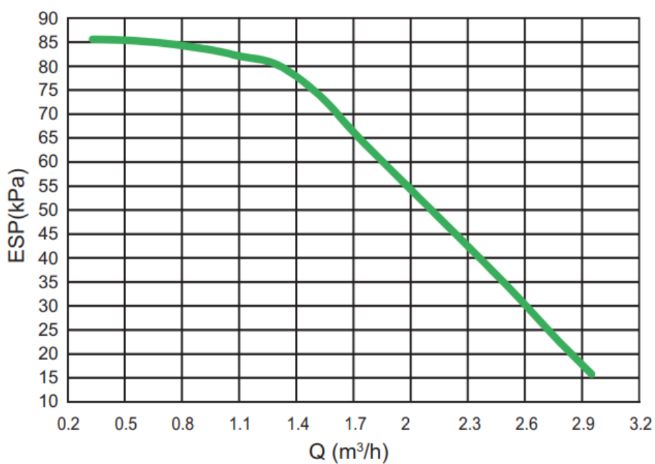
Čerpadlo WILO Para 25/9-87/IPWM1
